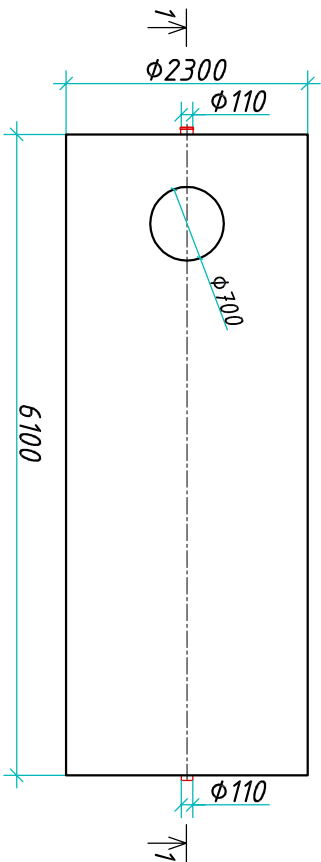
Вид сверху
